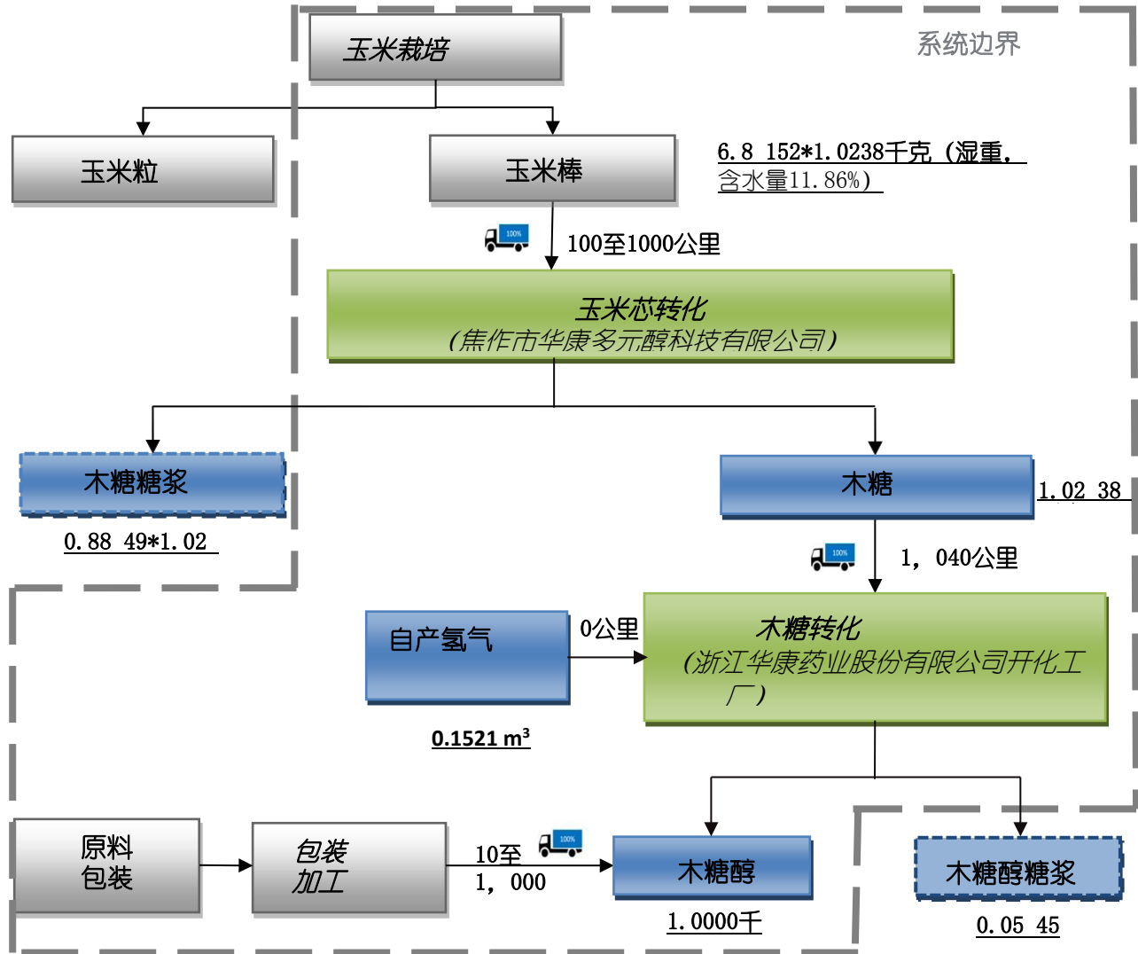
图III-1: 工艺流程图
