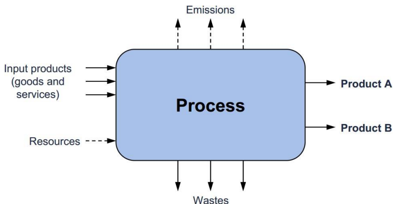
图III-3：消耗多种投入产品和资源以及产生各种废物和排放的多功能工艺（来源：ILCD手册）
